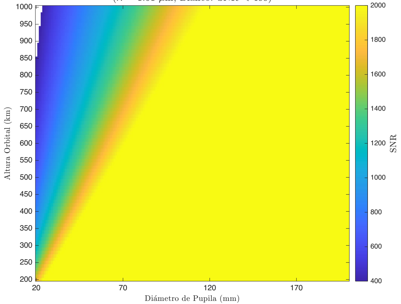
SNR - Korsch - Detector 2 ( \lambda = 1.61 \mu\text{m} , Blanco: SNR < 400)
